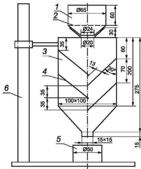
1 — воронка; 2 — защитная сетка № 1,6; 3 — корпус из прозрачного органического стекла; 4 — наклонные стеклянные пластины; 5 — цилиндрический стакан вместимостью (100 \pm 0,05) см 3 ; 6 — стойка
