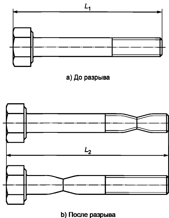
Рисунок 8 — Определение удлинения после разрыва A
