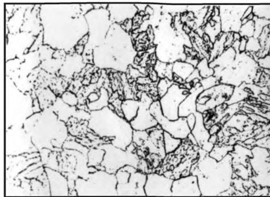
Балл 3, 500 x , химическое травление
