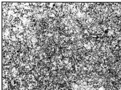
Балл 1, 100 x , химическое травление
