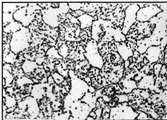
Балл 3, 500 x , электролитическое травление
