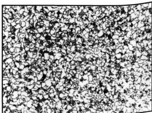
Балл 4, 100 x , химическое травление
