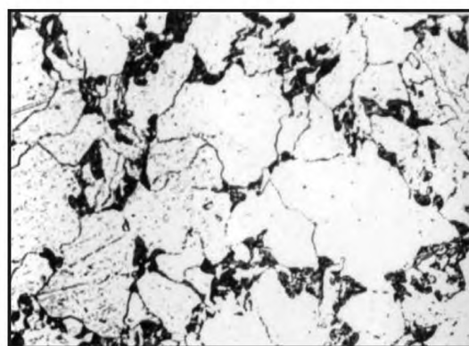
Балл 8, 500 x , электролитическое травление
