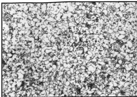
Балл 6, 100 x , химическое травление
