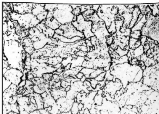
Балл 2, 500 x , химическое травление
