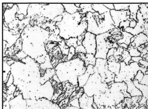
Балл 5, 500 x , химическое травление
