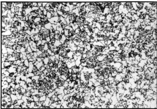
Балл 3, 100 x , химическое травление
