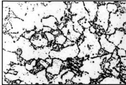
Балл 5, 500 x , электролитическое травление
