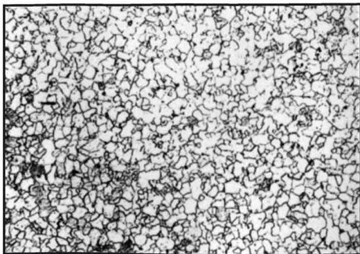
Балл 7, 100 x , химическое травление
