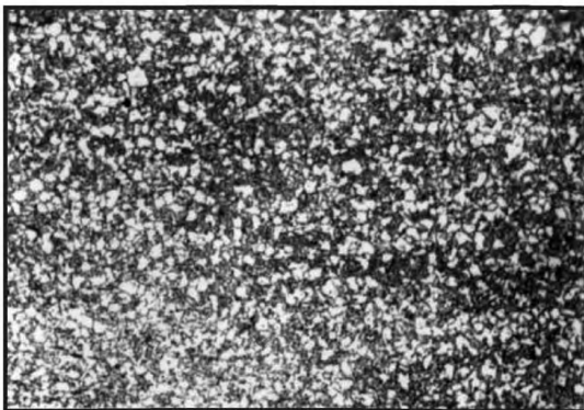
Балл 3, 100 x , электролитическое травление
