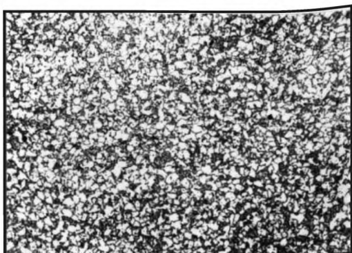
Балл 4, 100 x , электролитическое травление
