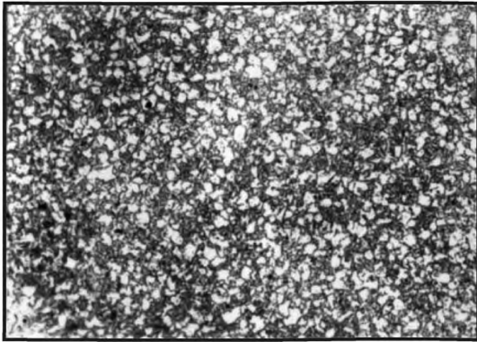
Балл 2, 100 x , электролитическое травление
