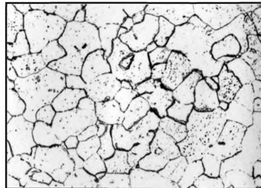
Балл 7, 500 x , химическое травление
