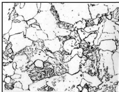
Балл 4, 500 x , химическое травление
