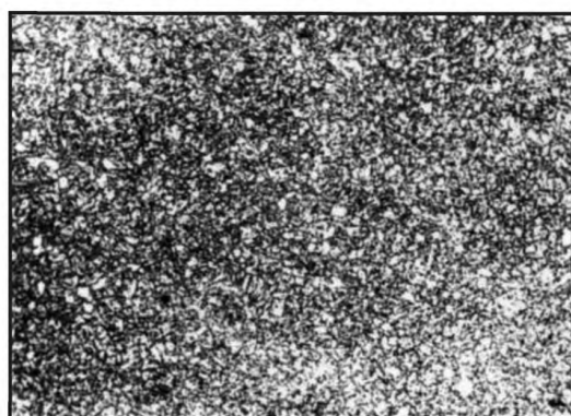
Балл 1, 100 x , электролитическое травление
