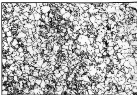
Балл 5, 100 x , химическое травление
