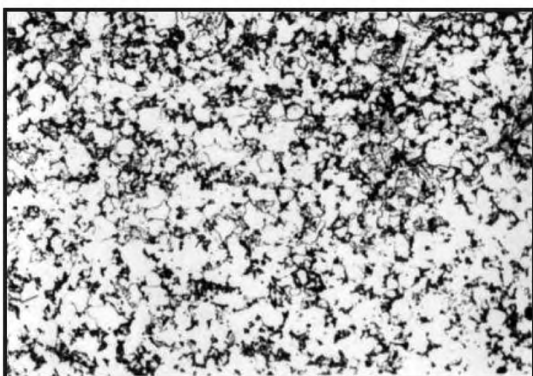
Балл 8, 100 x , электролитическое травление
