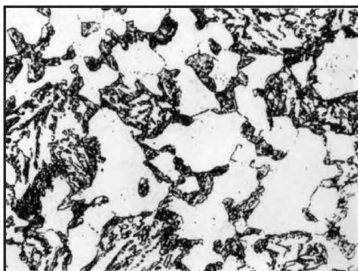
Балл 8, 500 x , химическое травление
