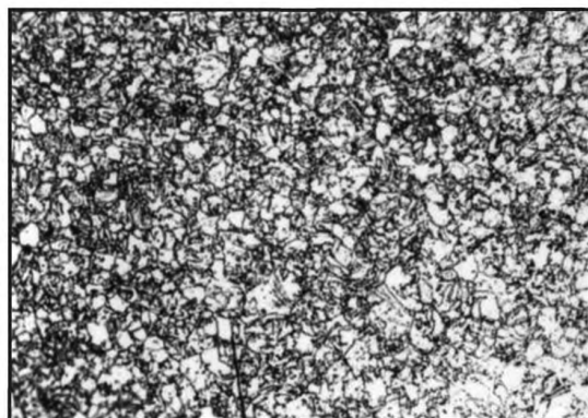
Балл 2, 100 x , химическое травление
