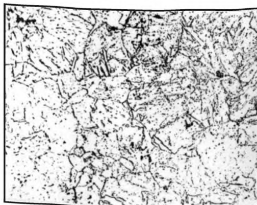
Балл 1, 500 x , химическое травление
