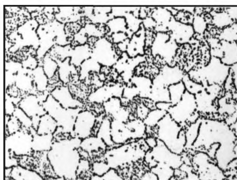
Балл 4, 500 x , электролитическое травление
