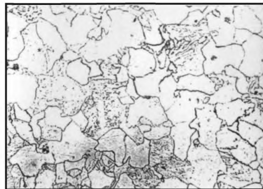
Балл 6, 500 x , химическое травление
