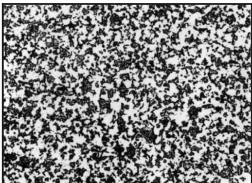
Балл 8, 100 x , химическое травление
