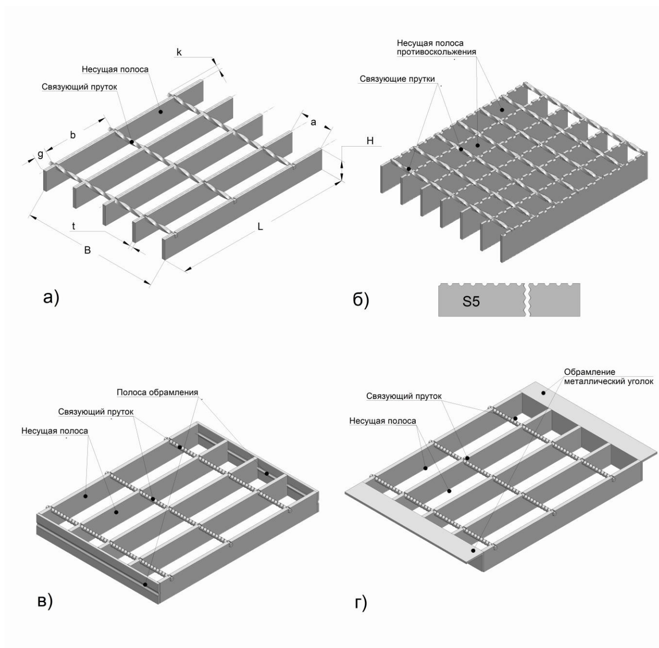
Рис. 1 Типовой вид сварного настила: а) без обрешетки со стандартной несущей полосой; б) без обрешетки с полосой противоскольжения; в) с полосой обрешетки; г) с уголком обрешетки.
