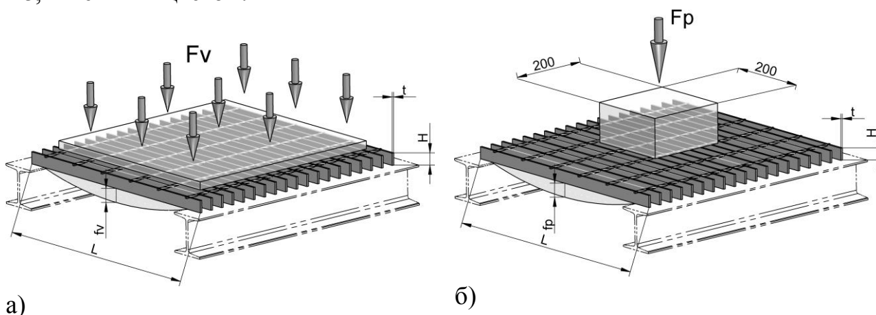
Рис. 3 Схема приложения к настилу равномерно распределенной нагрузки (а) и сосредоточенной нагрузки (б):
