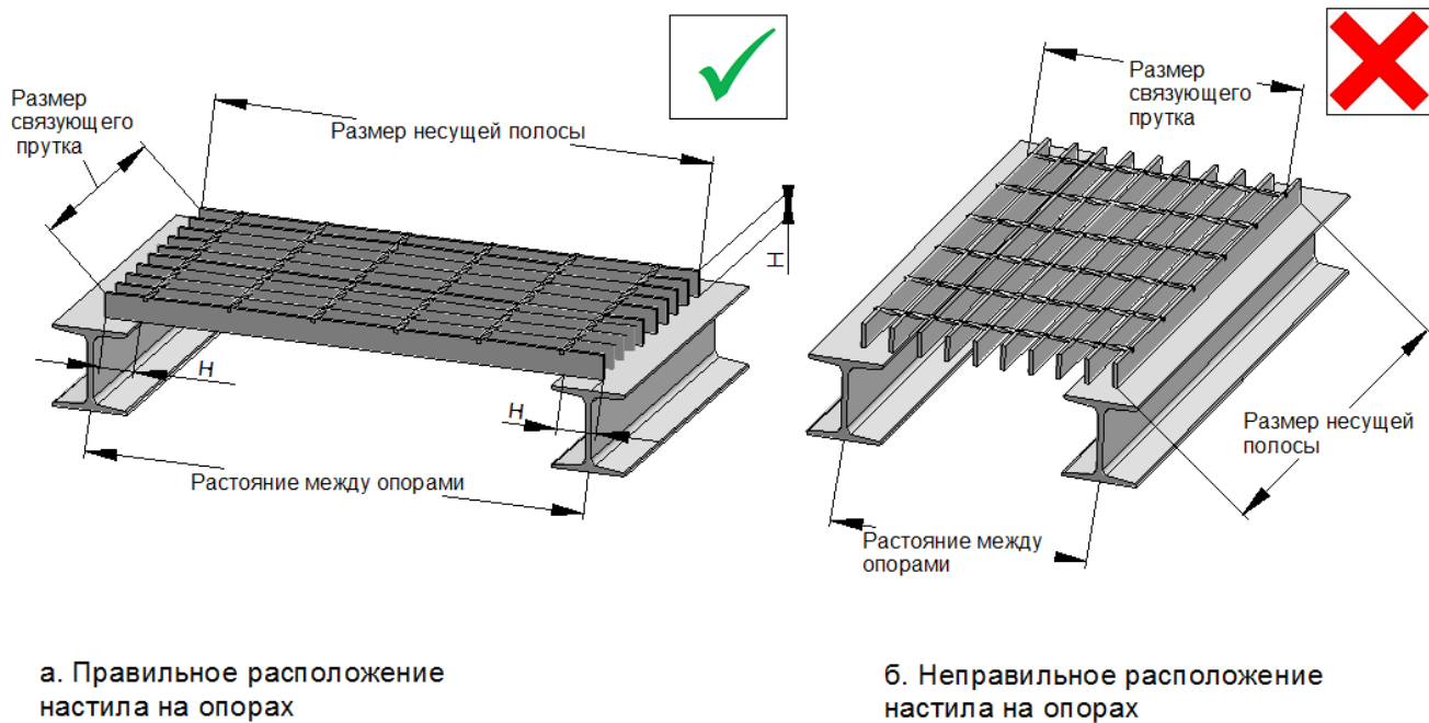
Рис. 4 Пример расположения настила на опорах:
